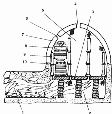
Secció d'un forn ceràmic d'època romana: 1. Praefurnium. 2. Cambra de foc. 3. Sòl. 4. Tir. 5. Cambra de cocció. 6. Observatori. 7. Volta. 8. Ceràmica. 9. Canals. 10. Falques aïllants.
