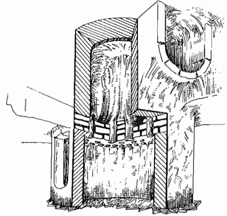
Form ibèrica d'Alcalá del Júcar, Albacete. Segle III a.C. Reconstrucció.
